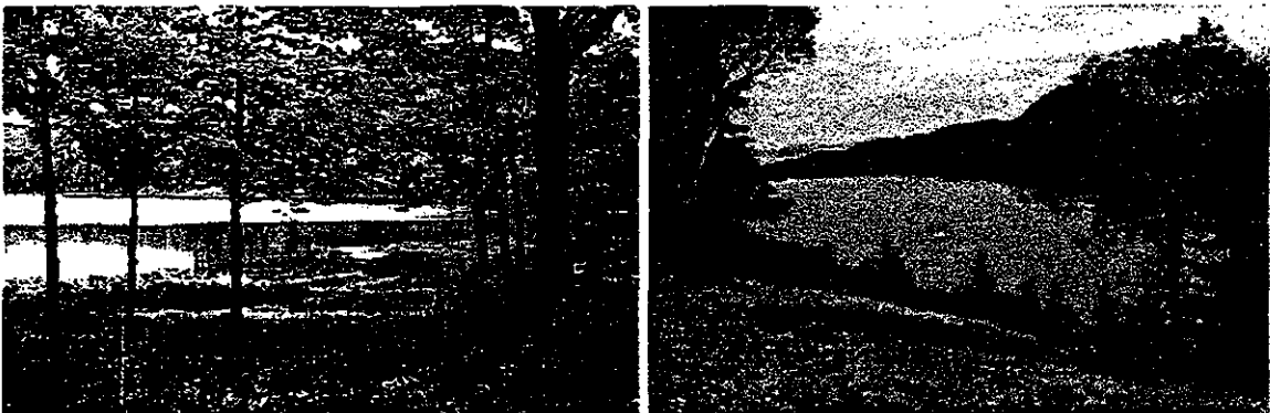
Fig. 3.8 – Floresta Temperada.
