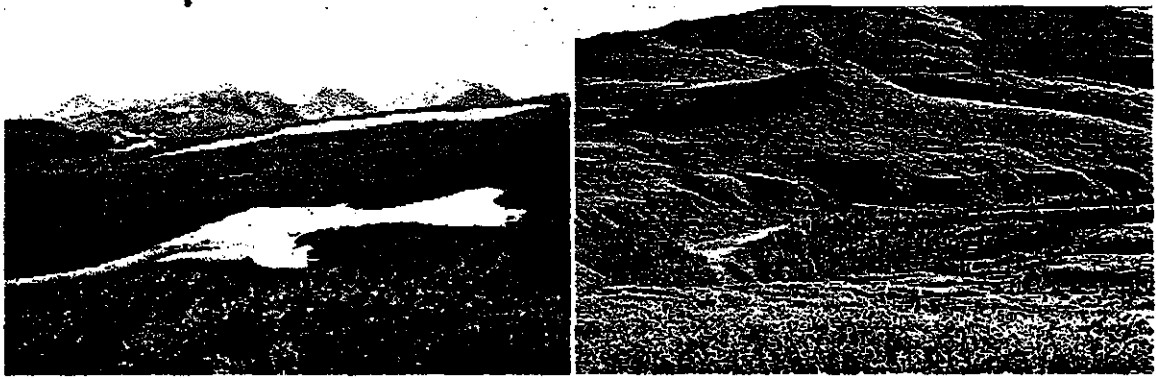
Fig. 3.6 - Tundra.
