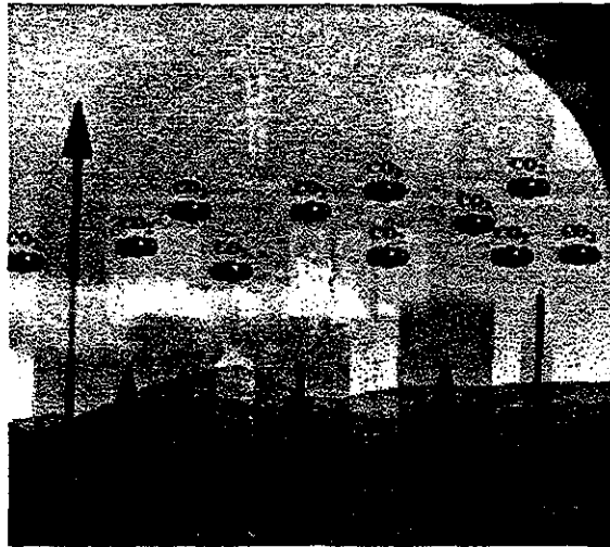
Fig. 5.6 – CO 2 absorvendo e refletindo radiação.
