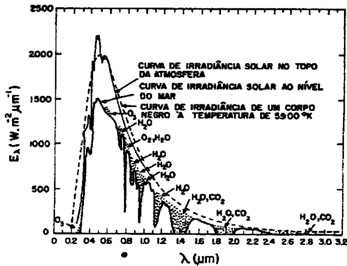
Fig. 2.1.4 - Intensidade de energia solar no topo da atmosfera na superfície terrestre e de um corpo negro a 6000° K.
