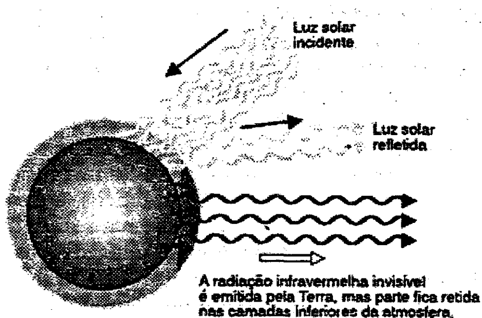
Fig.1 - Como atua o efeito estufa.
