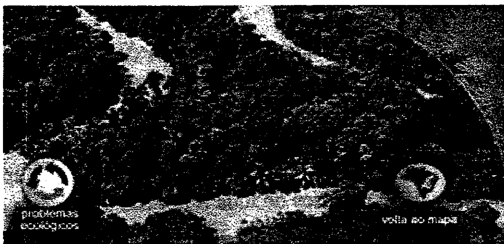
Fig. 3.14 – Floresta Amazônica.
