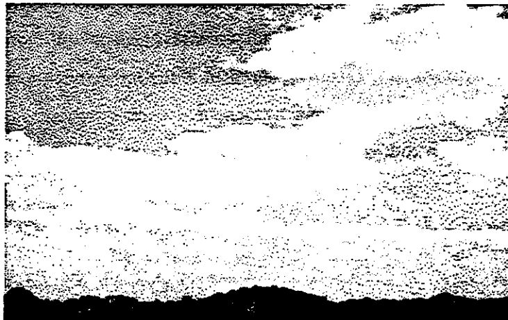
Fig. 7.3 – Cumulus humilis.
