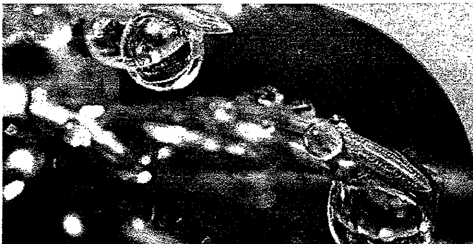
Fig. 7.11 - Orvalho.
