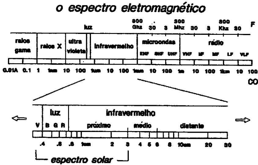
Fig. 2.1.3 - O espectro eletromagnético e suas principais regiões.
