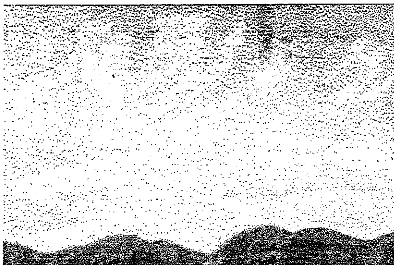
Fig. 7.6 – Cirrus uncinus.
