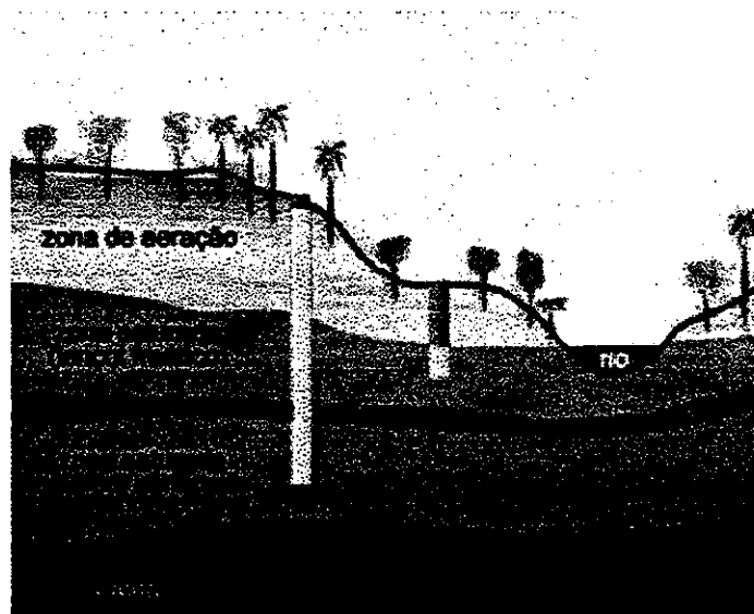
Fig. 2.19 – Divisões do solo.
