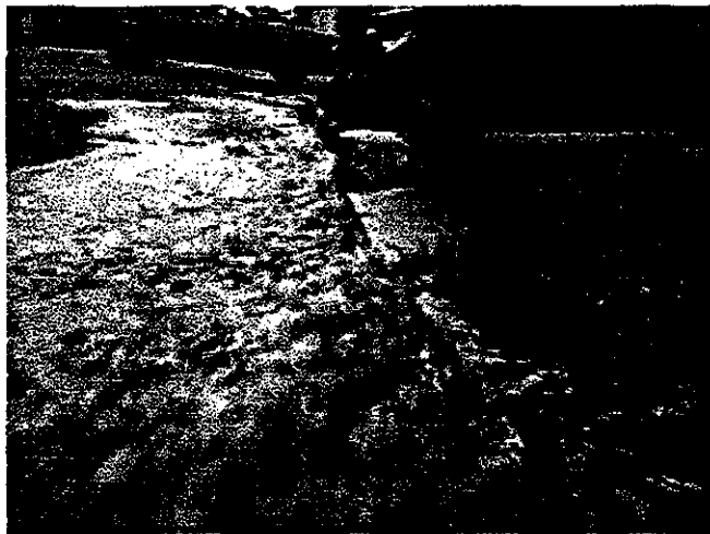
Fig. 2.14 - Enxurrada.
