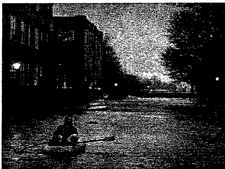
Fig. 2.20 - Enchente.
