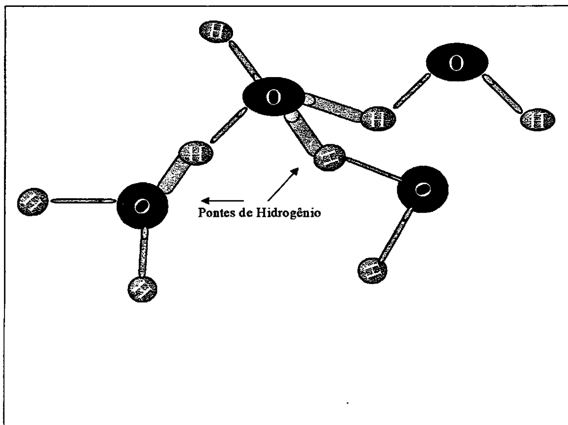
Fig. 3 – Pontes de Hidrogênio das Moléculas de Água
