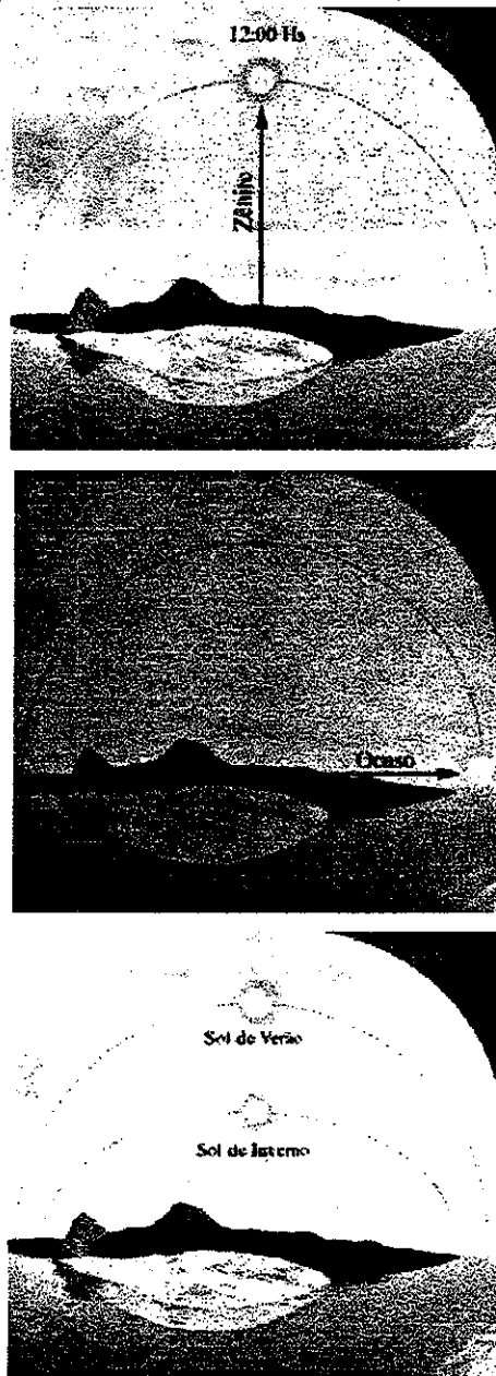
Fig. 5.3 – Posição relativa do Sol no céu.
