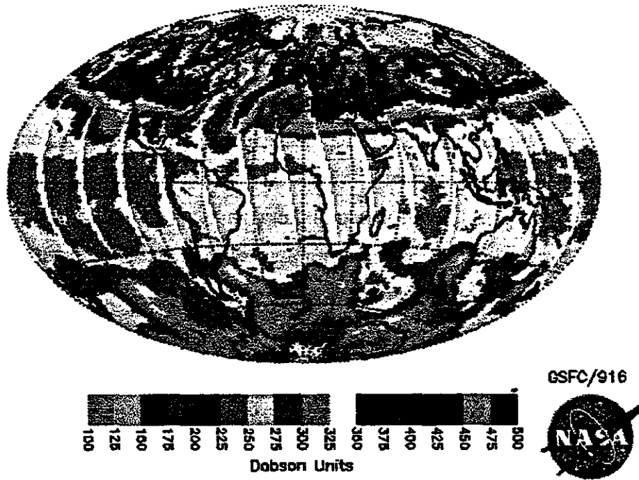
Fig. 8.3 - Coluna total de ozônio global medida pelo EP/TOMS para o dia 10 de março de 1998. Fonte: GSFC/NASA (2000)
